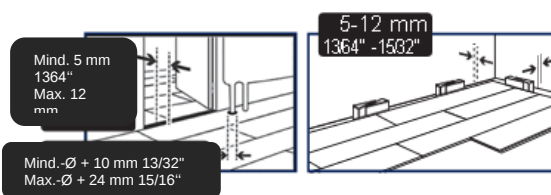
DEHNUNGSFUGE
